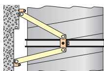
Gaine circulaire fixée à une paroi avec décrochement
