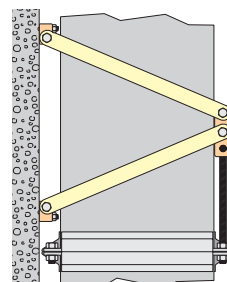
Gaine rectangulaire suspendue à la console par des tiges filetées
