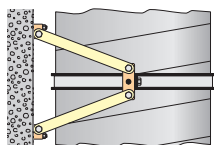
Gaine circulaire fixée à un mur plan
